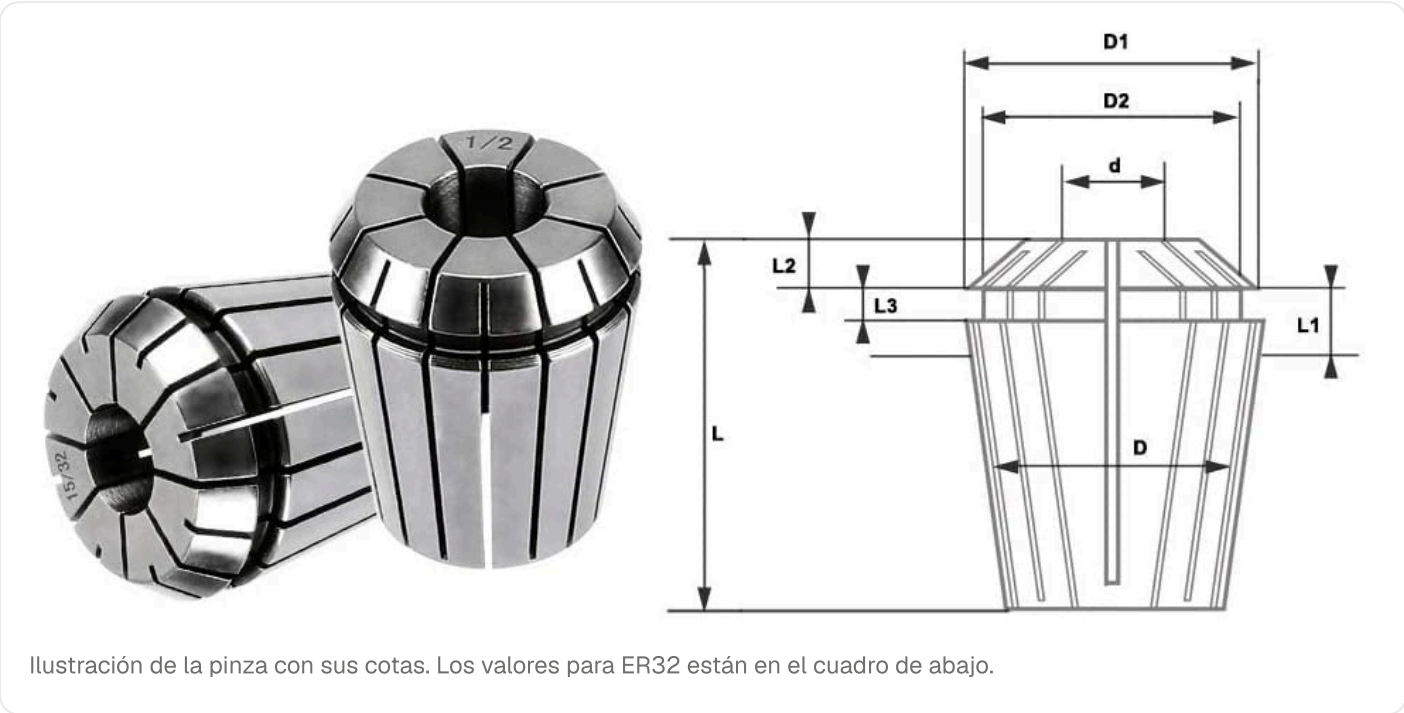
Cotas de la pinza ER32
